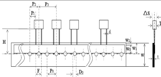
Fig.2 P=10.0、15.0mm
